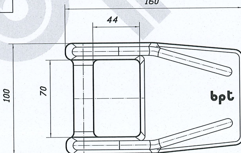
CERNIERA SOTTOSOPRA PER RIBALTABILE
